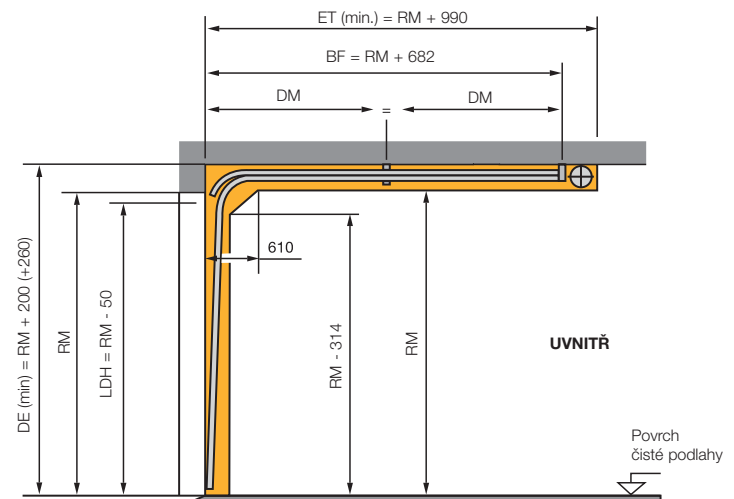
Kování L
